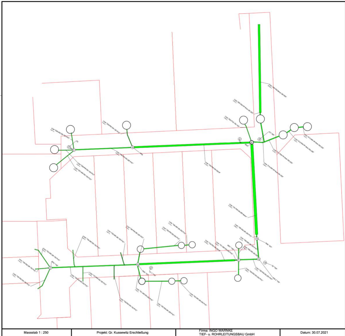
Abb2. Ausführungsplanung der Regenwasserrückhaltung und -ableitung (Fa. Ingo Warnke, Tief- und Rohrleitungsbau)
