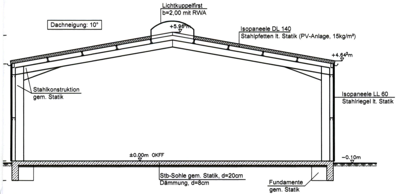
Schnitt A-A
